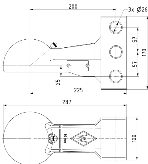
Spojovací hlavice ZKK80-157
