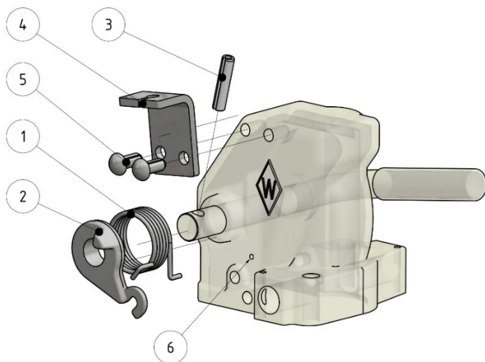
Afbeelding 1: Ombouwset FB 2000
