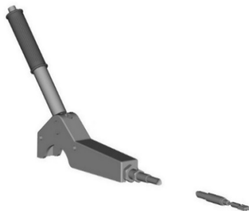
2. ábra: Karos bowden huzal
