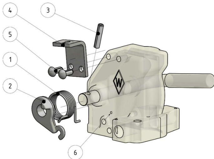
1. ábra: FB 2000 utólagos felszerelő készlet
