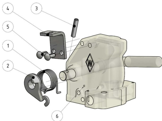
Figur 1: Eftermonteringskit FB 2000
