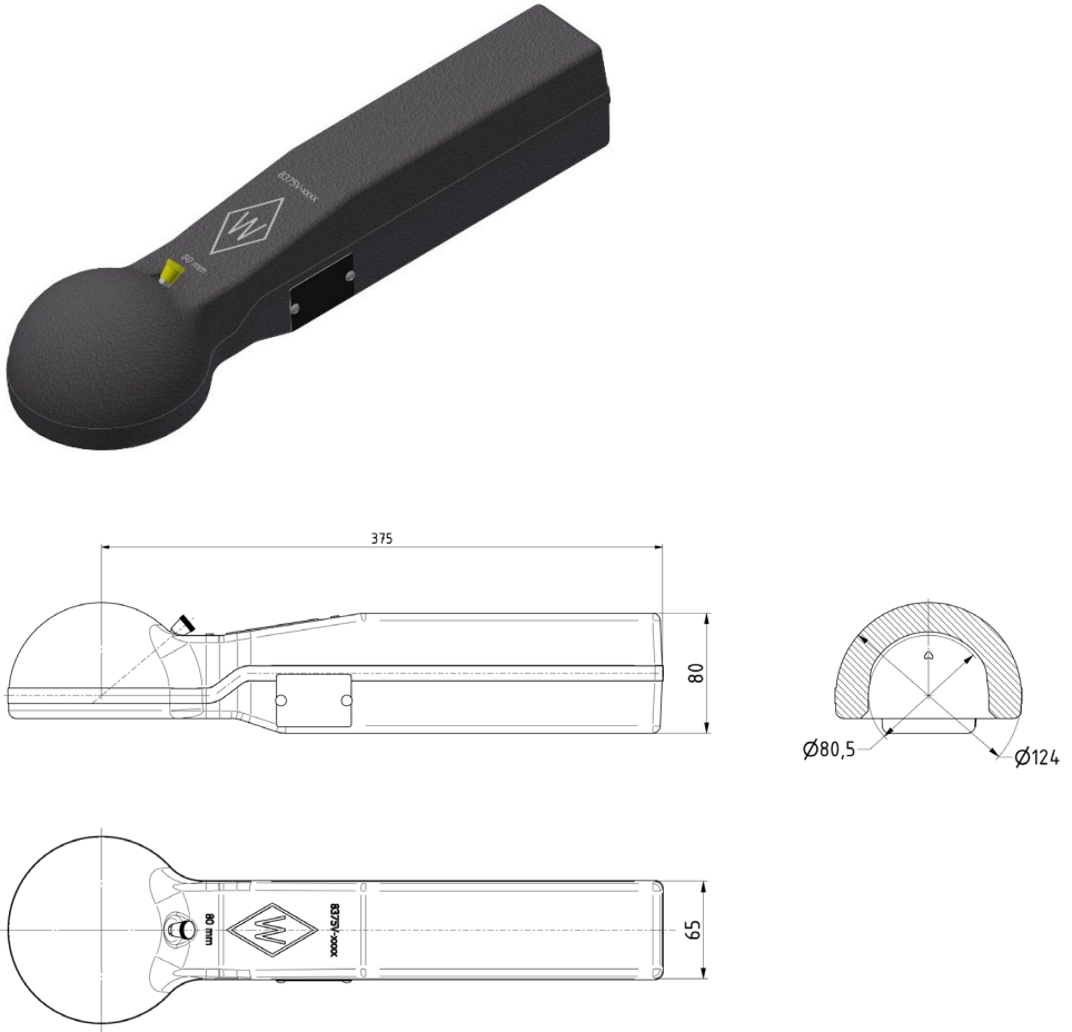
ZKK80-375V kapcsolófej
