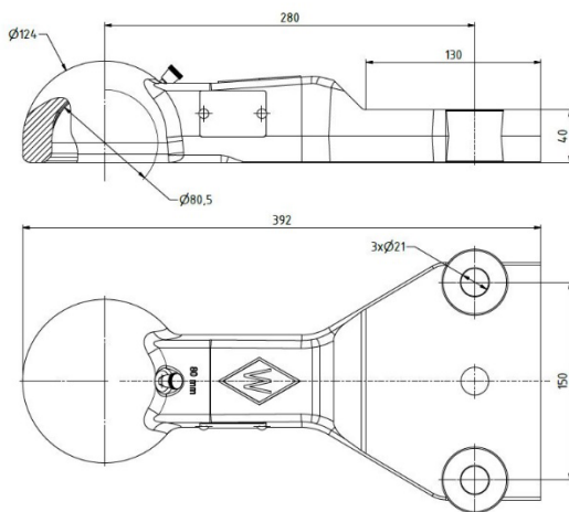
Kopplingshuvud ZKK80-150
