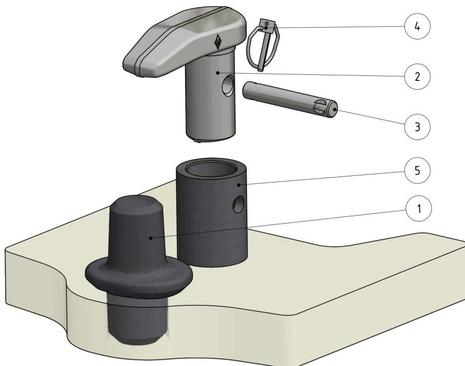
Pirštinis fiksatorius su pasukamu fiksatoriumi
