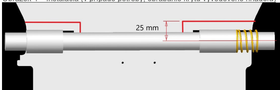
Obrázok 4 – Inštalácia (v prípade potreby, obrábanie krytu vývodového hriadeľa)
