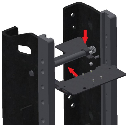
Obrázok 3 – Inštalácia
