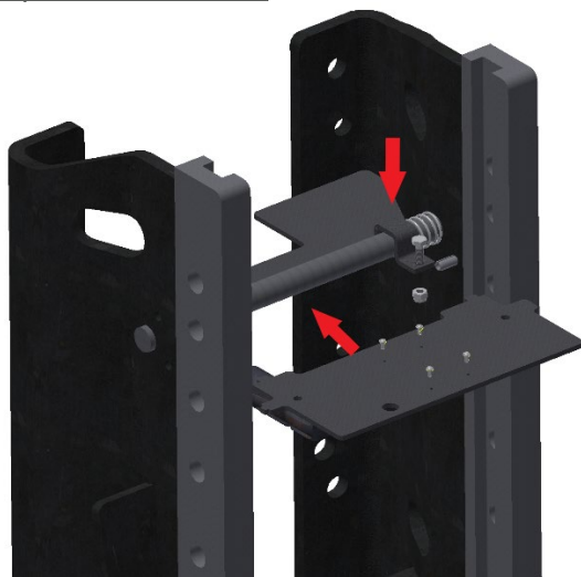
3 pav. – Montavimas
