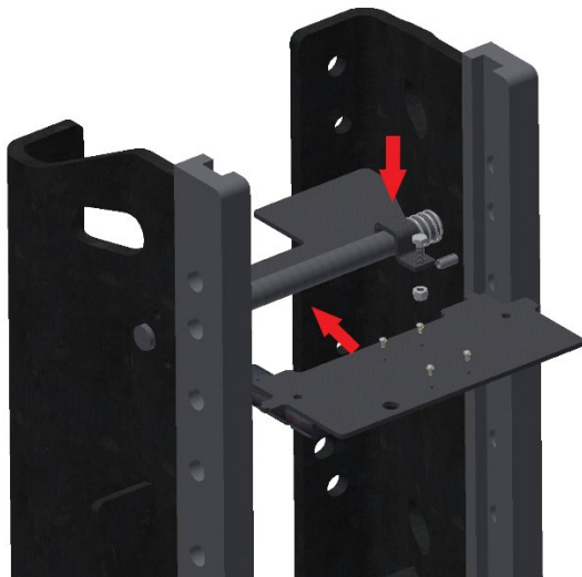
3. attēls – Uzstādīšana
