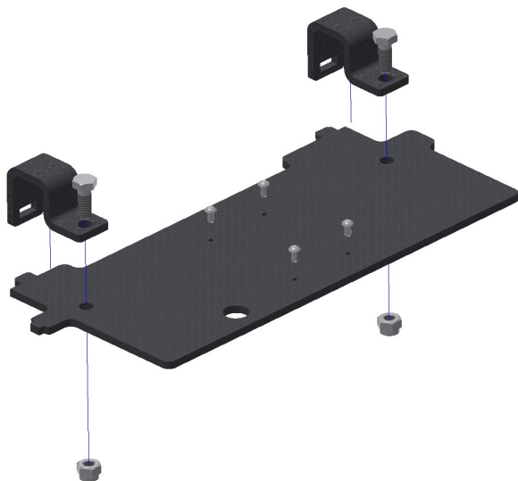
2. attēls – Uzstādīšana
