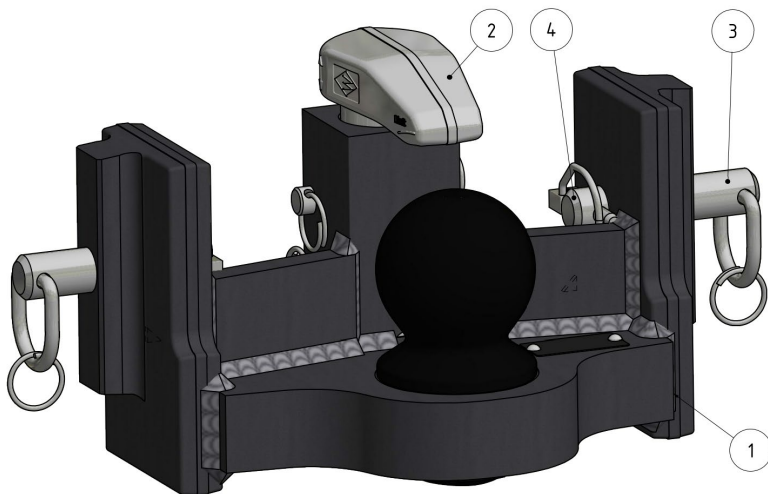
Kuulakytkin KB 8322
