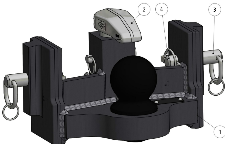
Kugleformet kobling KB 8322
