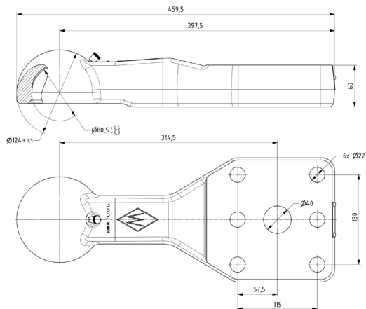
Kogelkoppeling ZKK80-115
