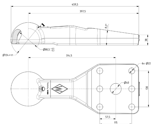
Kogelkoppeling ZKK80-115W
